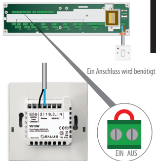
An WW-Timer angeschlossener Zylinderthermostat
