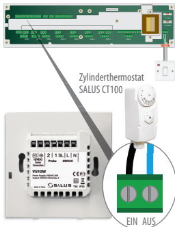
An Klemmleiste angeschlossener Zylinderthermostat (Standard)
